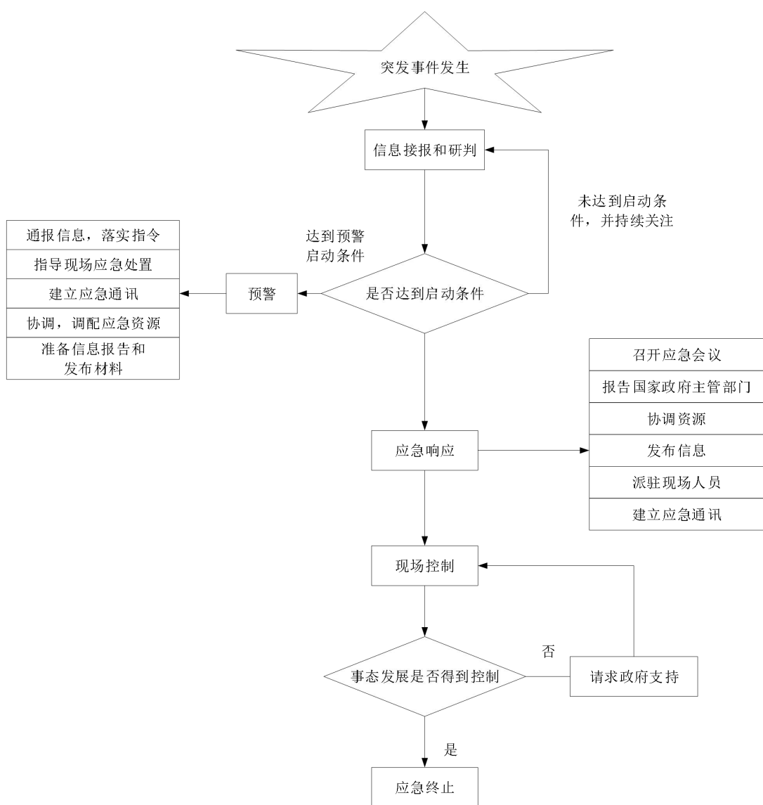
图 3-2 突发环境事件应急响应流程图
